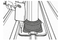
5. Rohrmanschette mit Schrauben oder Bulbbitte Niete befestigen
