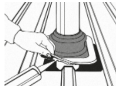
3. Dichtungsmasse auftragen
