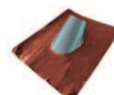
Dachdurchführung „Eco Green“ 22°-42° Elastomere / Bleiersatz Terrakotta
